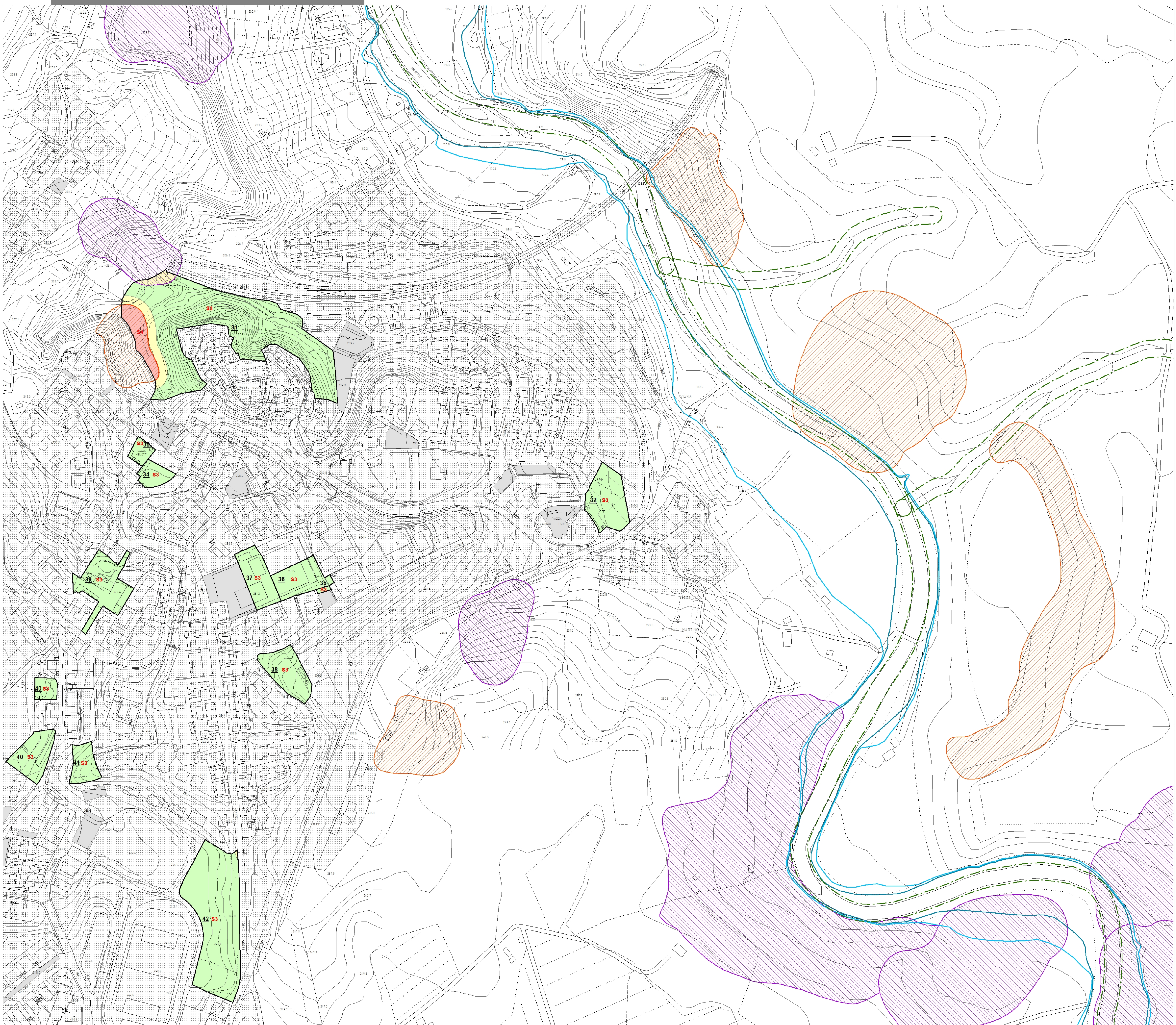
Carta delle fattibilità (geologica, sismica, idraulica) scala 1:2.000
